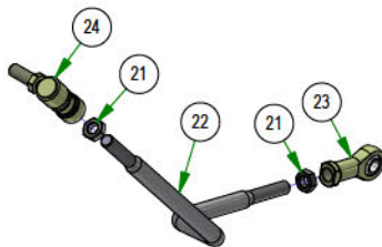
035-5450-00 Push Rod-Right
